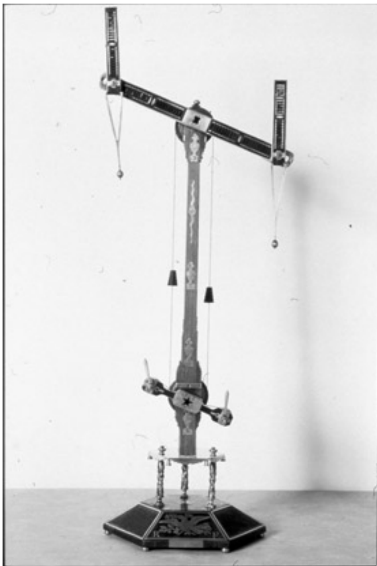
Ci-contre : Maquette du télégraphe aérien conservée par Mathieu Durant, directeur à Saint-Malo. © Musée de la Poste
